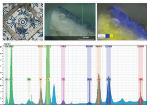
圖 2-1-11 · 研發群組「臺灣本業敷瓦的文化資產價值探討及材料特性分析」臺南廳長官邸壓印染付花紋敷瓦元素分布圖及X光螢光光譜（國立臺北藝術大學）
