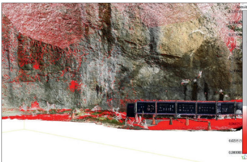
圖 5-2-1 · 國定考古遺址八仙洞考古遺址（靈岩洞左側）地貌變異監測比對結果（紅色區域為疑似有變動區域）
