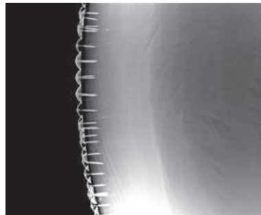
圖 5-2-6 · 獨木大鼓之金屬鉚釘X光影像
