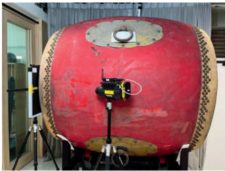
圖 5-2-5 · 獨木大鼓之X光檢測儀器設置
