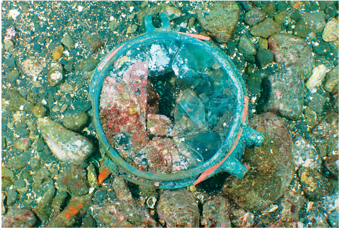
圖 3-5-13 · 山藤丸 2022 年度監看作業新發現船窗，有助瞭解其沉船結構
