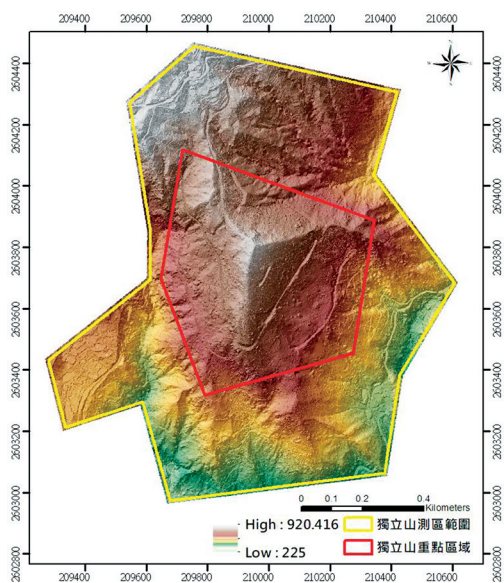
圖 5-1-1 · 阿里山林業暨鐵道文化景觀獨立山螺旋登山鐵道場域調查成果 (DEM)
