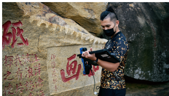
圖 5-2-1 · 碑碣 3D 掃描作業現況
