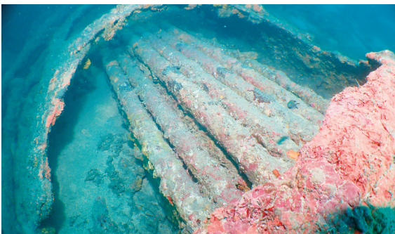
圖 3-5-4、圖 3-5-5 · 「外淺石 1 號」經調查具有蘇格蘭鍋爐特徵
