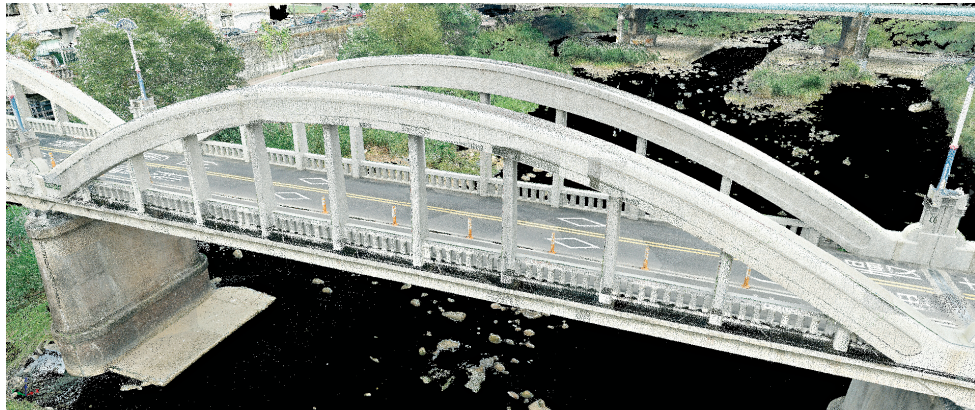
圖 2-1-8·研發群組「古蹟橋梁檢測與監測管理系統」：三峽拱橋光達掃描（財團法人國家實驗研究院國家地震工程研究中心）
