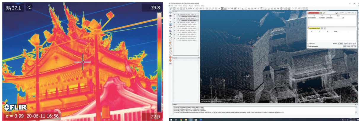
▶ 圖2-1-9 · 文化資產學院研發群組「國定古蹟北港朝天宮預防性保存之室內外環境檢視與模擬解析」計畫以熱影像找尋問題區域
