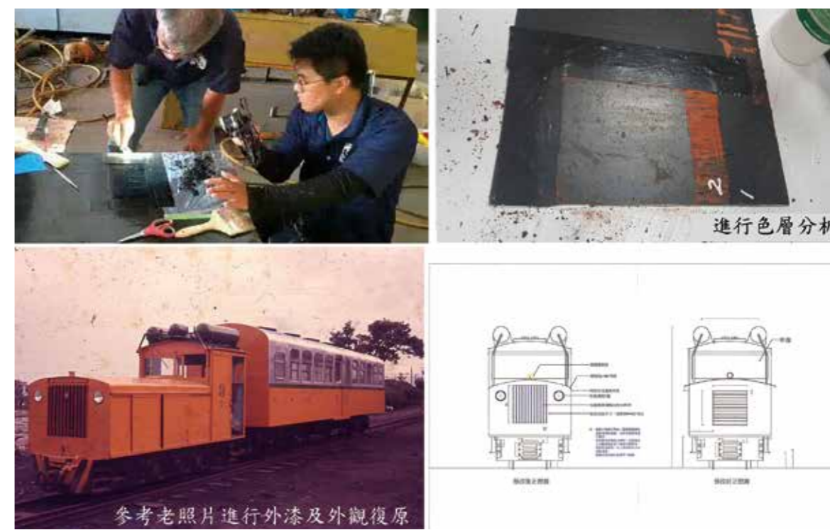
圖2-3-20 · 羅東林場七噸柴油車修復考究準備工作
