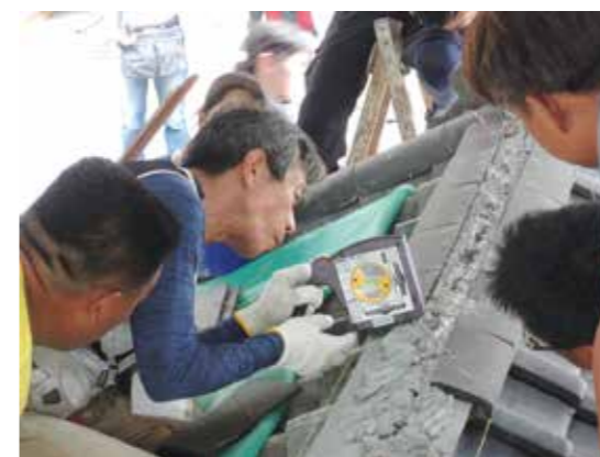
圖4-3-7 日本匠師使用勾配定規檢測屋脊熨斗瓦斜率
