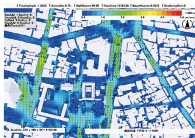
圖2-1-6·文化資產學院研發群組「台南市孔廟周邊區域保存環境模擬與對策分析」計畫，透過CFD模擬出熱季晚上時段風場分布
