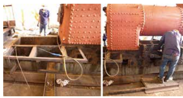
圖2-3-22 · 羅東林場15號蒸汽火車施工
